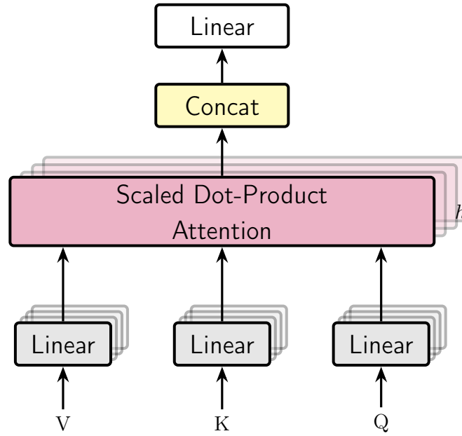
Figura 3.1: Diagrama de la atención multi-cabeza
