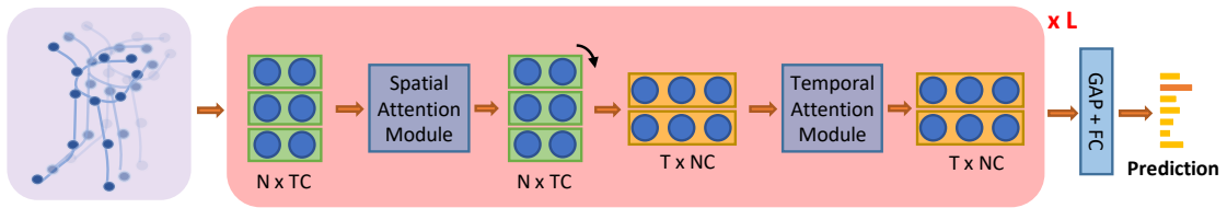
Figura 3.8: Esquema de la red. Obtenido de [35]
