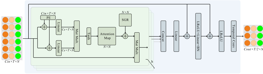
Figura 4.4: Esquema del módulo de atención de keypoints del cuerpo. Se toma h = 6 . Imagen de [19]
