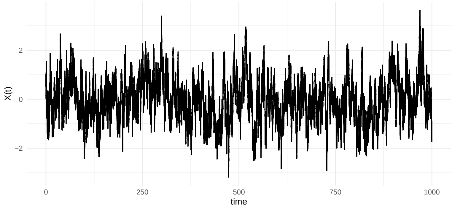
OU covariate path
