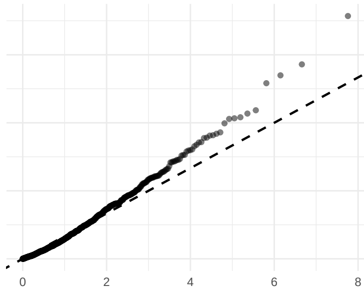
Poisson_wrong
