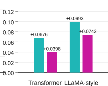
Brecha de generalización (gap)
