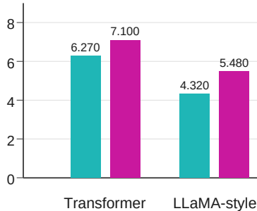
Perplejidad (PPL)
