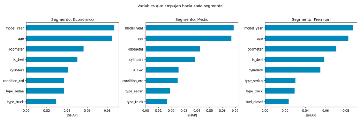
Figura 8. Variables que empujan la clasificación hacia cada segmento de precio.
