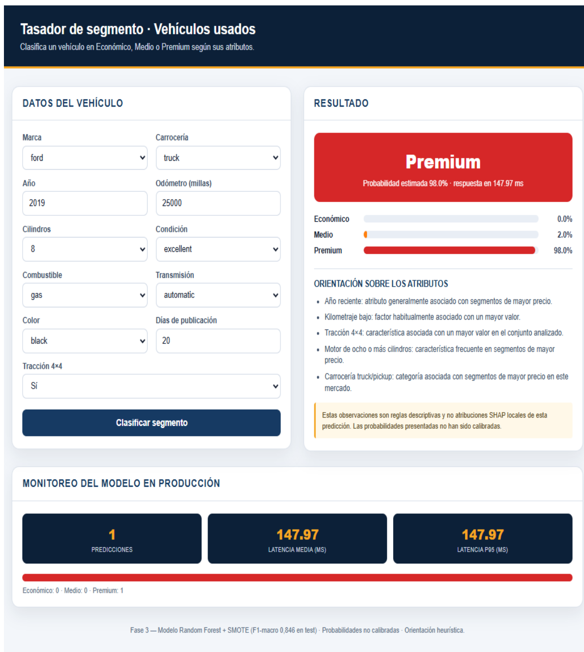
Figura 5. Interfaz del sistema mostrando una predicción, sus probabilidades estimadas, la orientación heurística y el panel de monitoreo.
