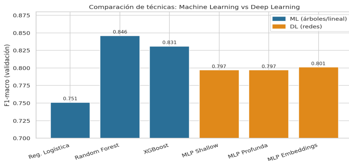
Figura 2. Comparación de F1-macro entre técnicas de Machine Learning y Deep Learning.
