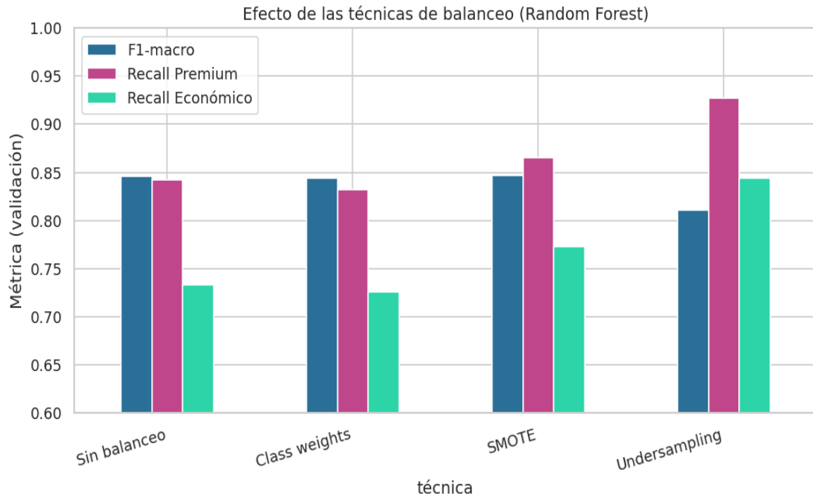
Figura 4. Efecto de las técnicas de balanceo sobre el desempeño del Random Forest.
