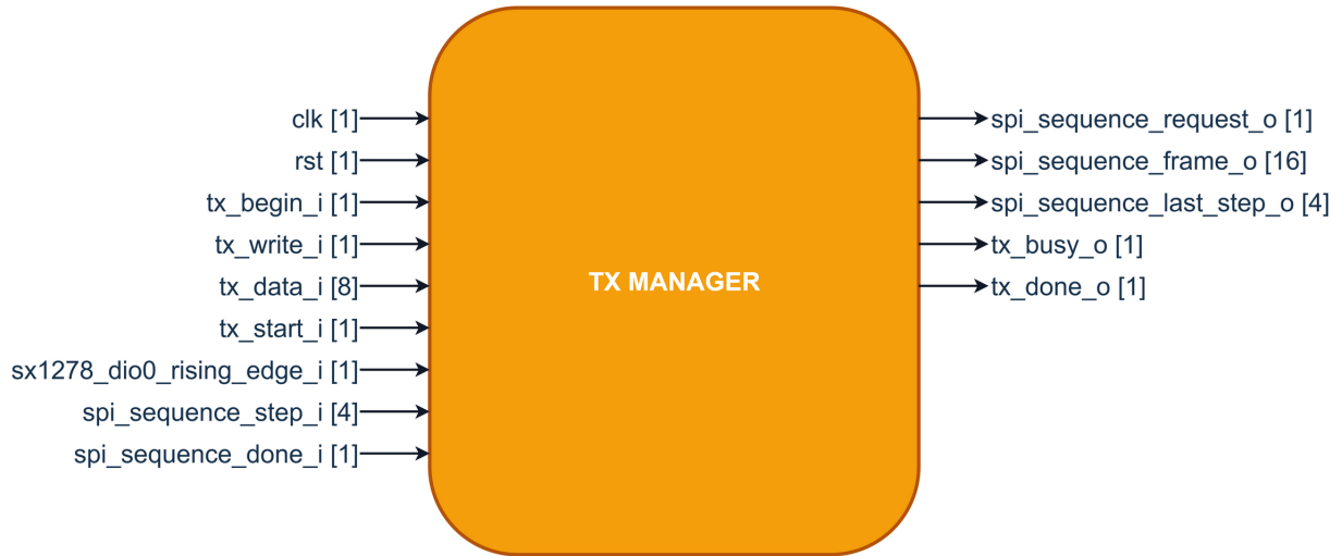
Figura 4: Entradas y salidas del manager de transmisión.
