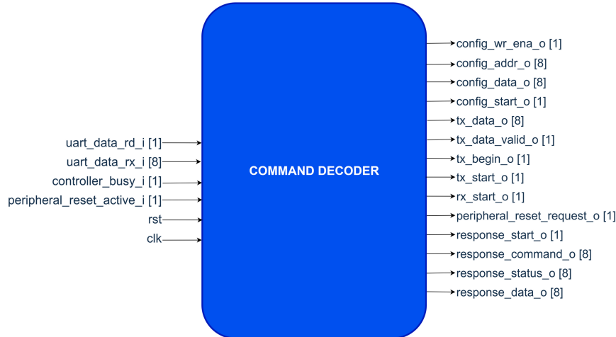
Figura 2: Interfaz del decoder de comandos UART.
