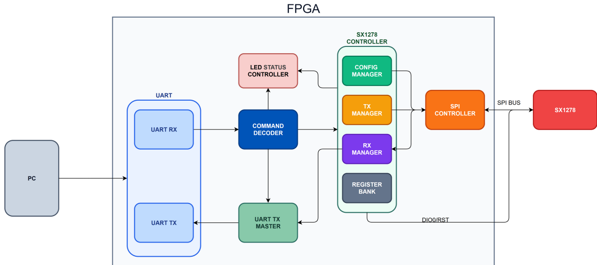
Figura 1: Diagrama en bloques del sistema completo.
