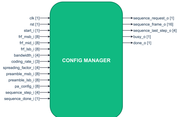
Figura 3: Entradas y salidas del manager de configuración.
