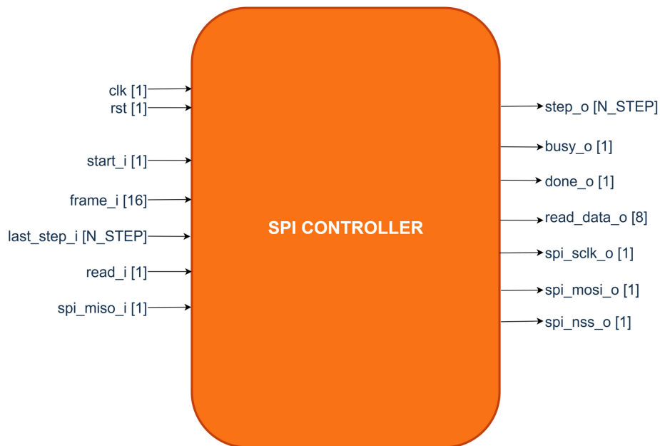
Figura 6: Interfaz del controlador de secuencias SPI.
