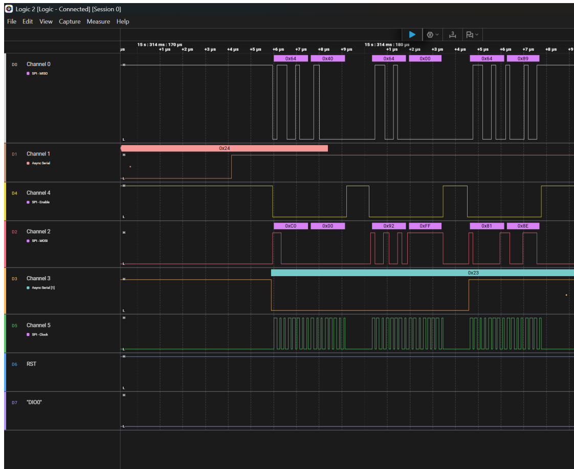
Figura 9: Configuración de DIO0, limpieza de IRQ e ingreso al modo RX.
