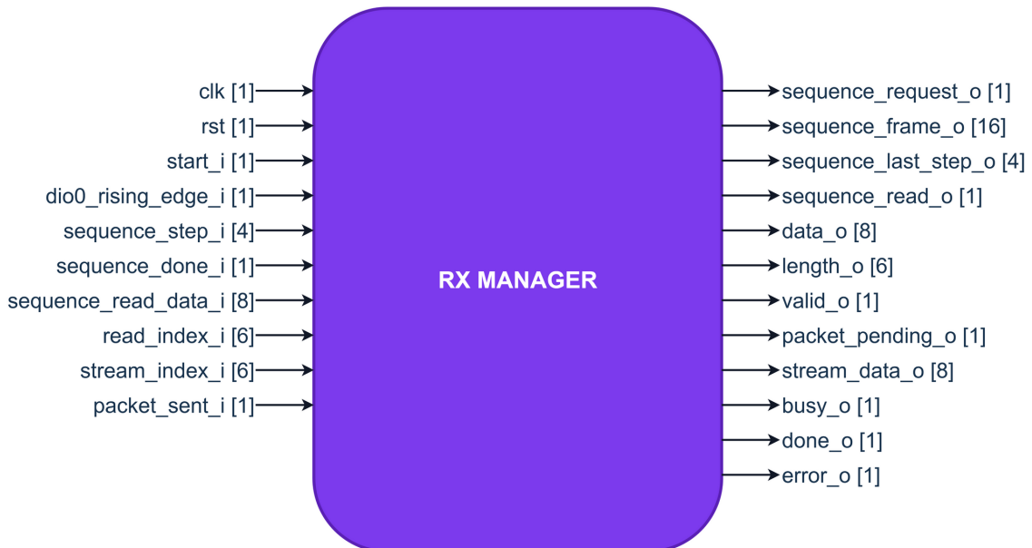
Figura 5: Entradas y salidas del manager de recepción.
