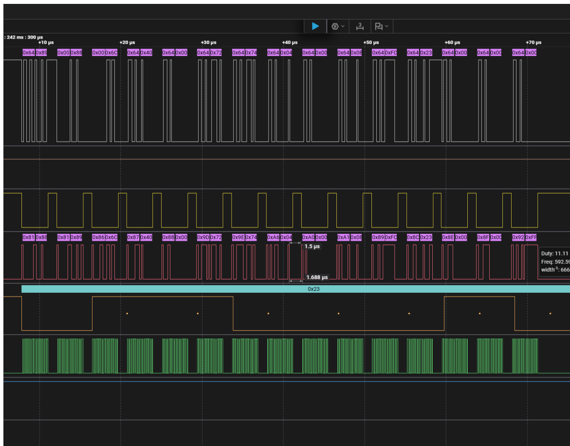
Figura 8: Secuencia SPI de configuración observada en hardware.
