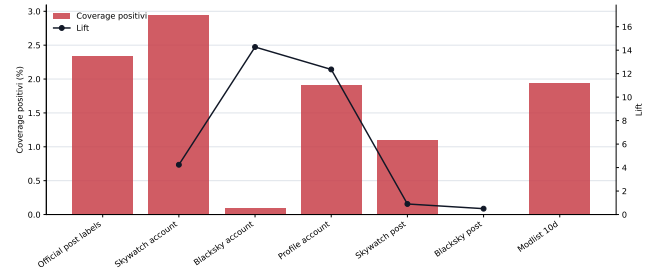
Figura 13: Coverage e lift per labels, labeler terzi e modlist. Il lift elevato di alcuni segnali non compensa la bassa coverage.
