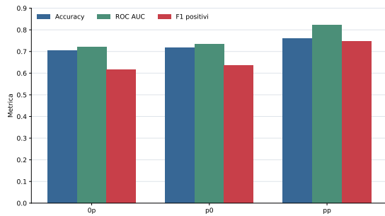
Figura 11: Performance held-out del modello principale per corner esposto.
