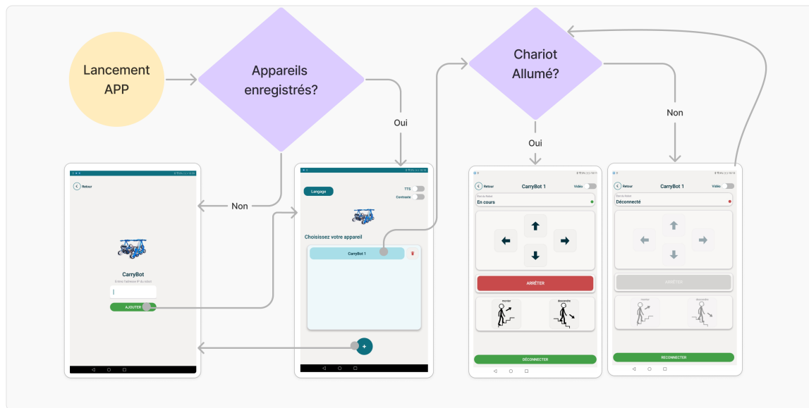
Diagramme de flux applicatif
