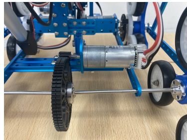
Illustration : ajout d'un second moteur arrière
