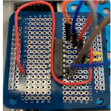
Illustration : ajout du pont en H L293D pour le vérin
