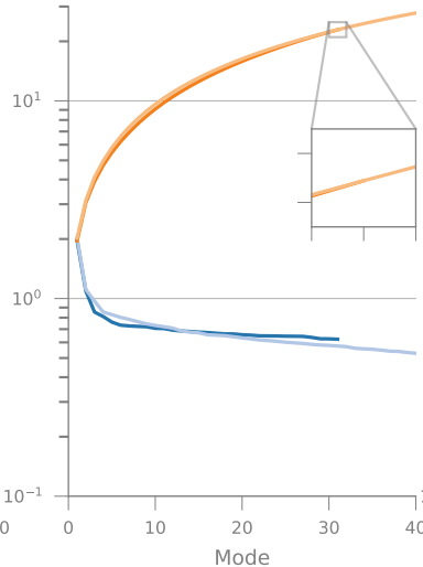
B | Singular Values \sigma
