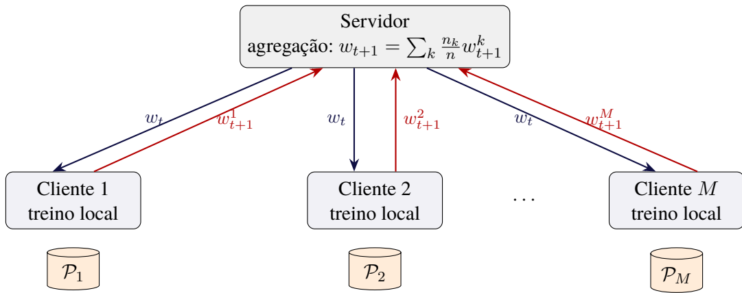
Figura 2.1 – Fluxo de uma rodada de aprendizado federado: o servidor distribui o modelo global (azul) e os clientes devolvem apenas atualizações ou gradientes (vermelho), mantendo os dados locais.
