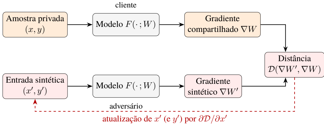
Figura 2.2 – Princípio dos ataques de inversão de gradientes baseados em otimização.
