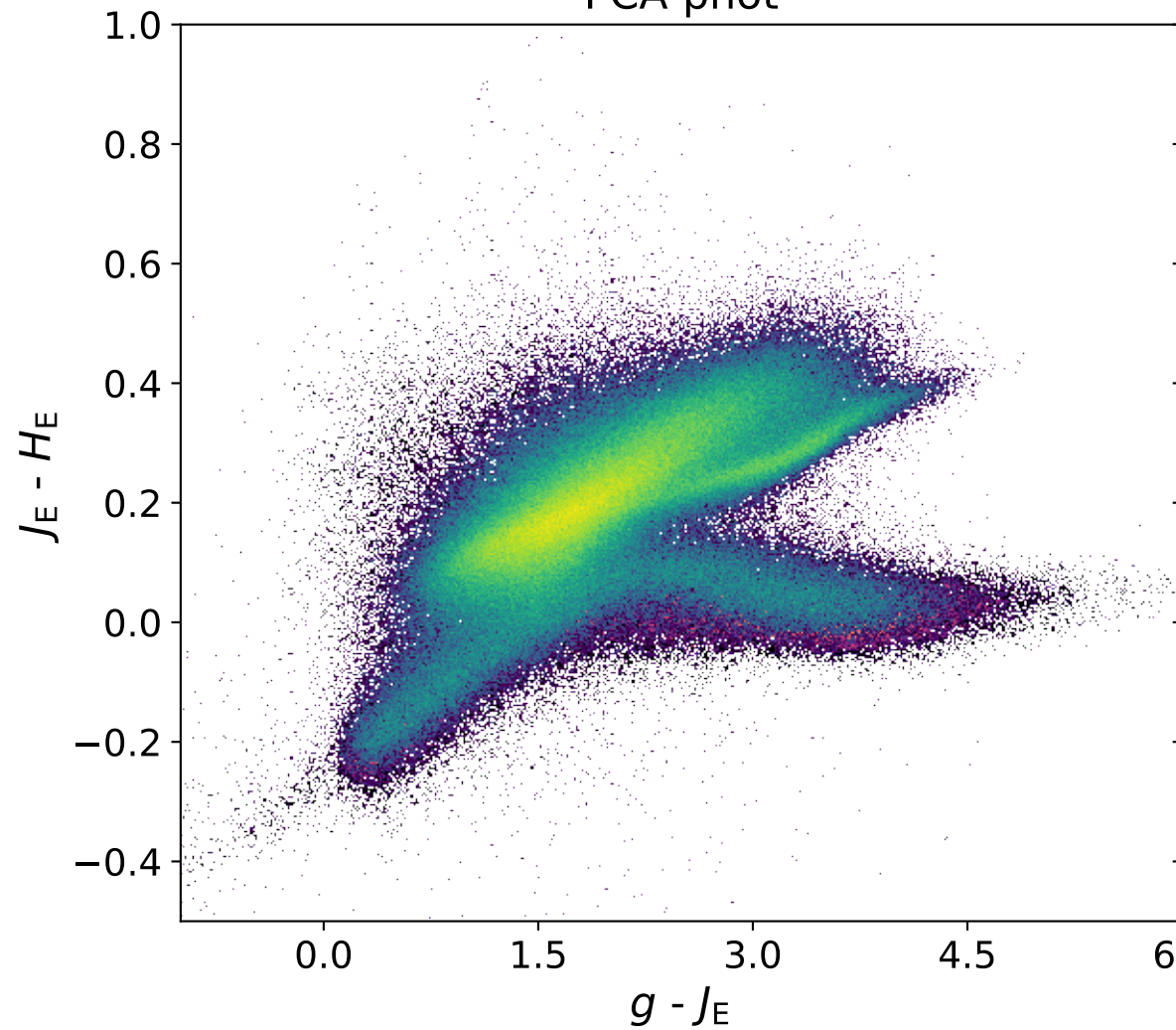
PCA-phot
