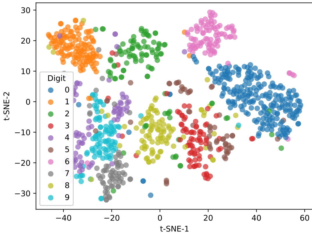
t-SNE
