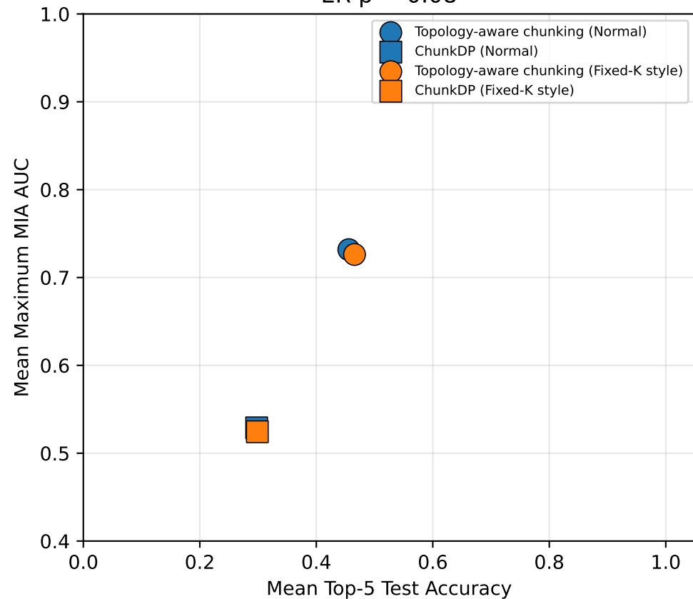
ER p = 0.08
