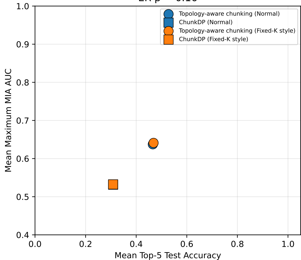
ER p = 0.16
