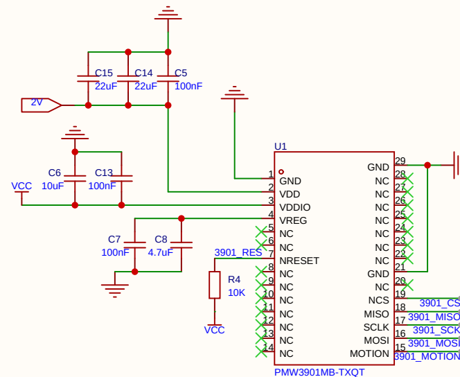
光流计
