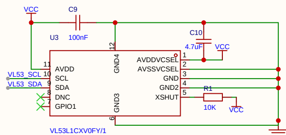
激光传感器
