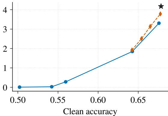
Citeseer
