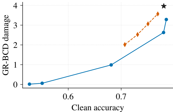
Cora
