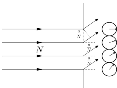
(a) 单缝衍射光路动画效果图
