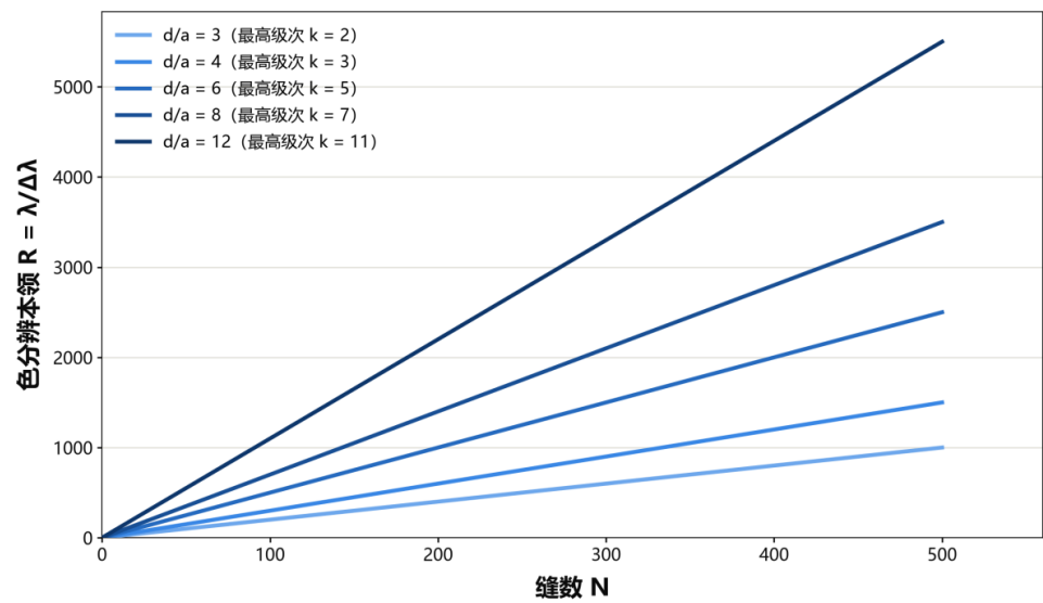
图 4: 考虑缺级：最高可用级次下的色分辨本领
