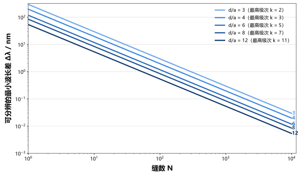
图 5: 可分辨的最小波长差随缝数的变化
