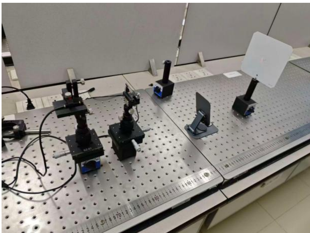
图 6: 实验装置图
