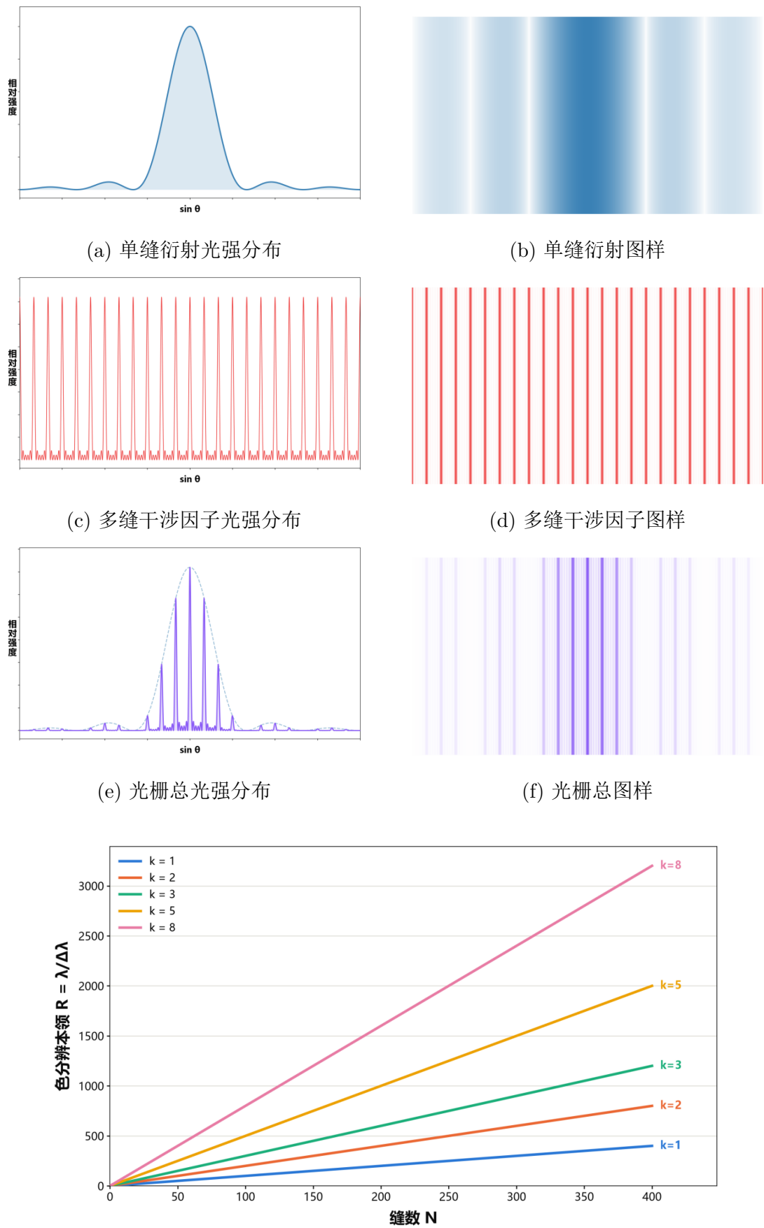
图 3: 光栅色分辨本领随缝数的变化
