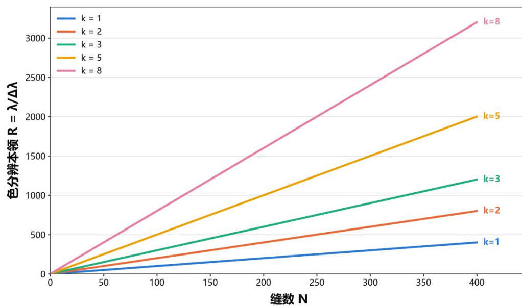
光栅色分辨本领随缝数的变化
