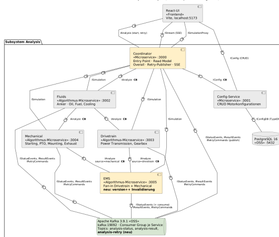
Bausteinsicht Ebene 2 - Whitebox Subsystem Analysis (UML-Komponentendiagramm)
