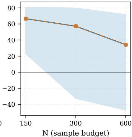
MuSiQue
