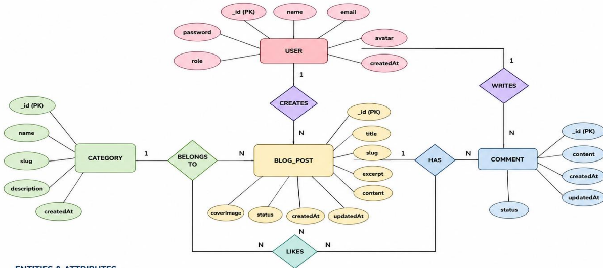
BlogNest – ER Diagram
