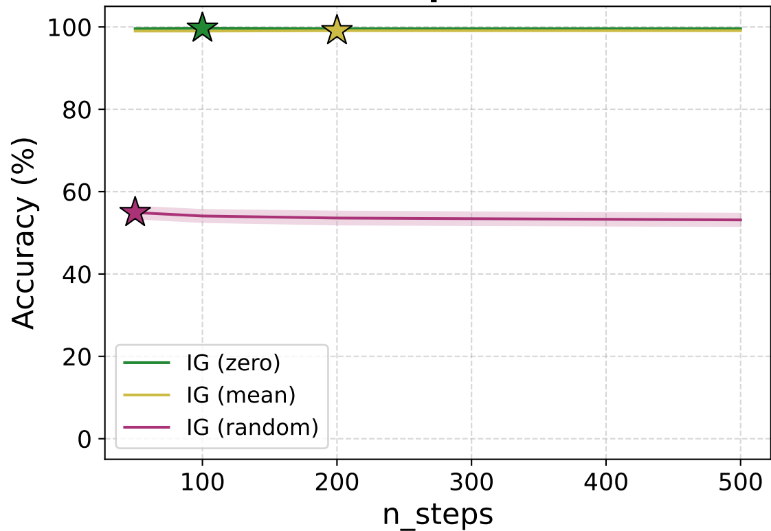
Top-2
