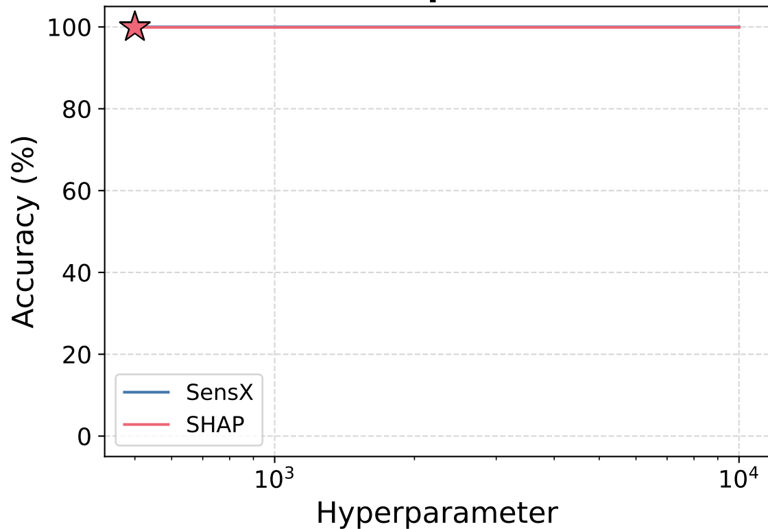
Top-2
