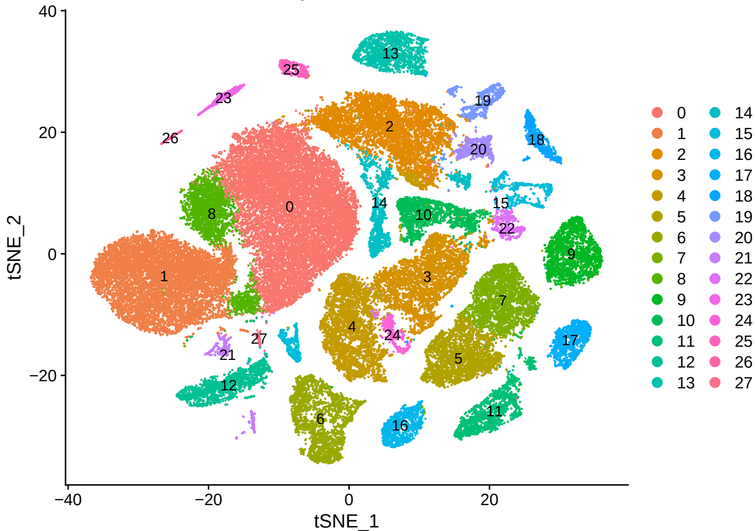
t-SNE by seurat_clusters
