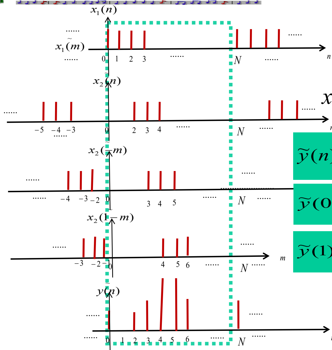
图 2-7 两个周期序列 ( N=7 ) 的周期卷积
