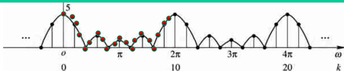
图 2-6 图2-3和图2-5的重叠图，它表明一个周期序列的DFS系数等于主值区序列的傅里叶变换的采样
