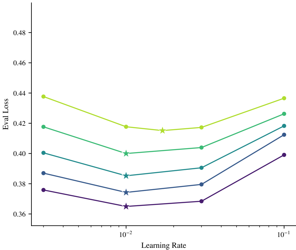
PoLoRA
