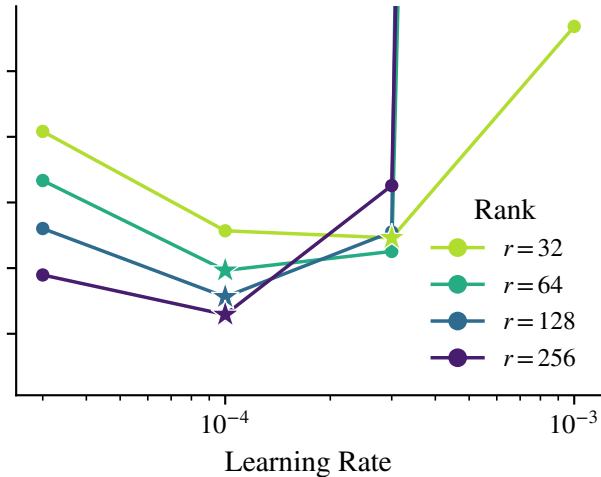
AdamW
