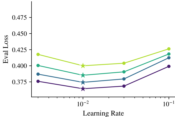
Polar-LoRA
