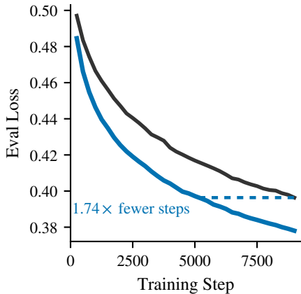
OLMo-2-1B
