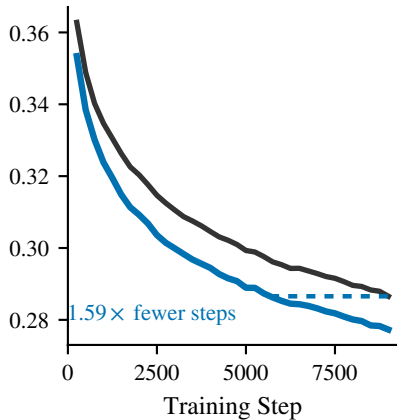
Llama-3-8B
