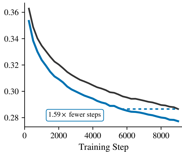
Llama-3-8B
