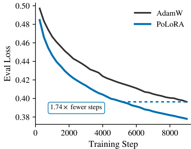
OLMo-2-1B
