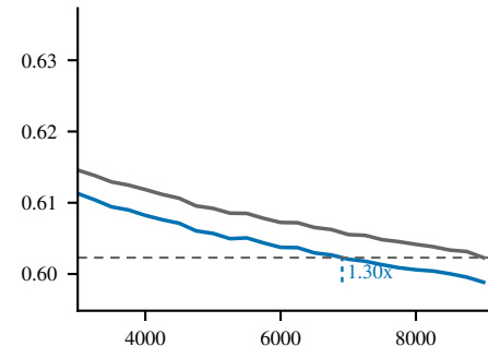
Qwen2.5-1.5B / opc-sft-stage2 / r=256
