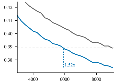
Llama-3.2-1B / OpenMathInstruct-2 / r=128
