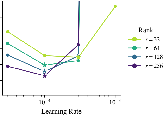
AdamW
