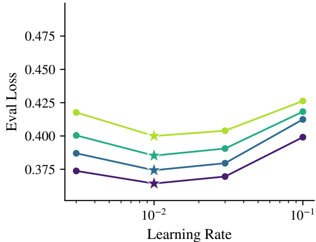
PoLoRA
