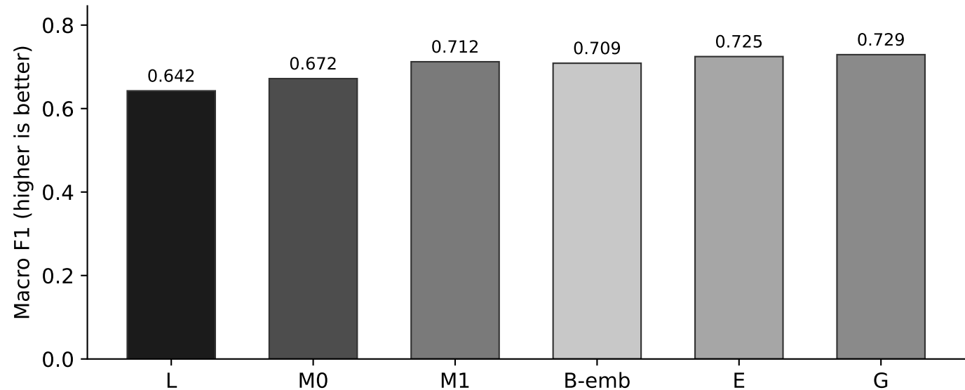
Canonical test set, N = 1331 - Macro F1
