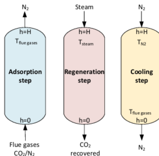
شکل 3 - چرخه در سه مرحله
