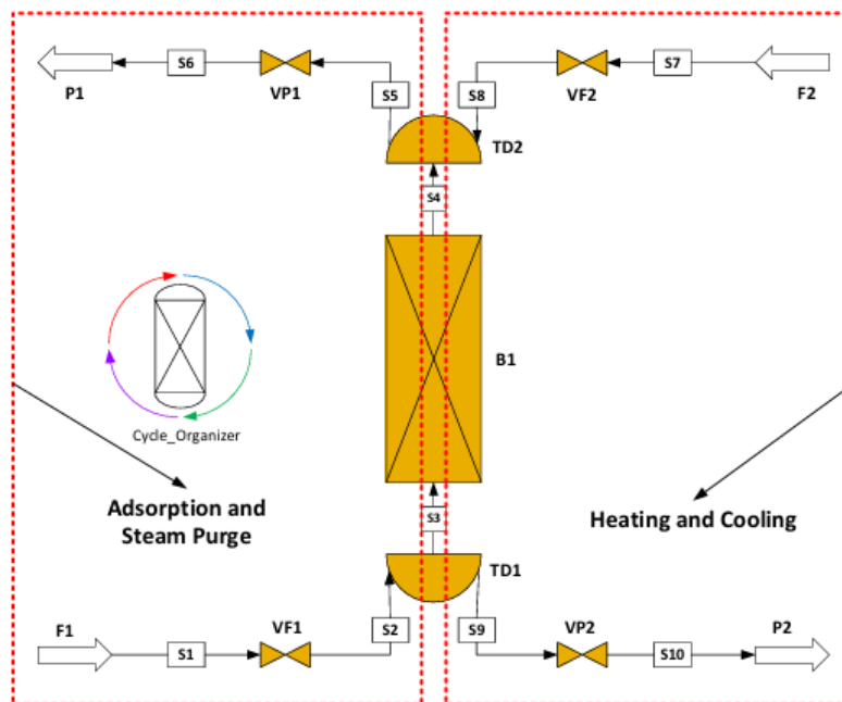
شکل 5 — 5 فلو شیت فرایند جذب در اسپن پلاس
