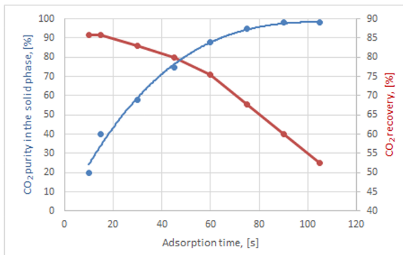
شکل 6 - خلوص و بازیابی \text{CO}_2 برای سیلیکاژل PEI
