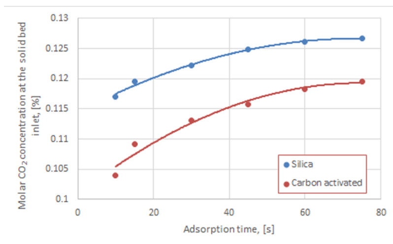
شکل 10 - غلظت \text{CO}_2 در بستر جاذب ها
