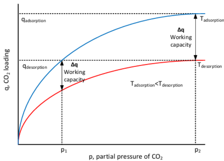
شکل 1- فرایند جذب نوسان دما
