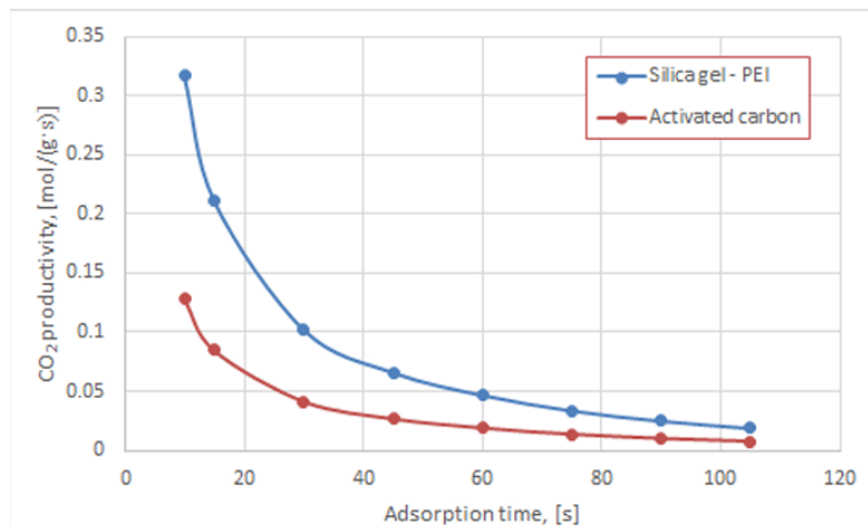
شکل 11 - بهره وری \text{CO}_2 با توجه به زمان جذب
