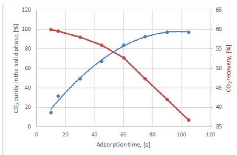
شکل 7 - خلوص و بازیابی \text{CO}_2 برای کربن فعال
