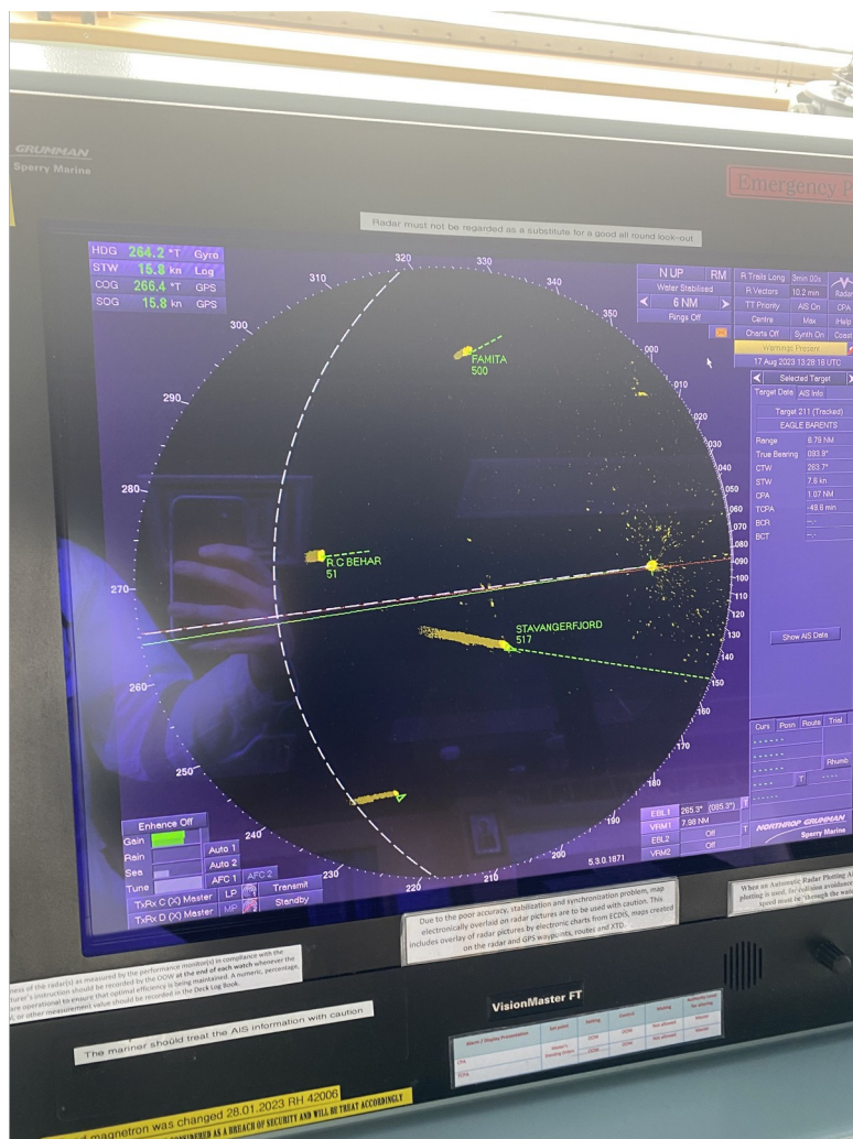
Рис. 3. Радар Sperry Marine VisionMaster FT
