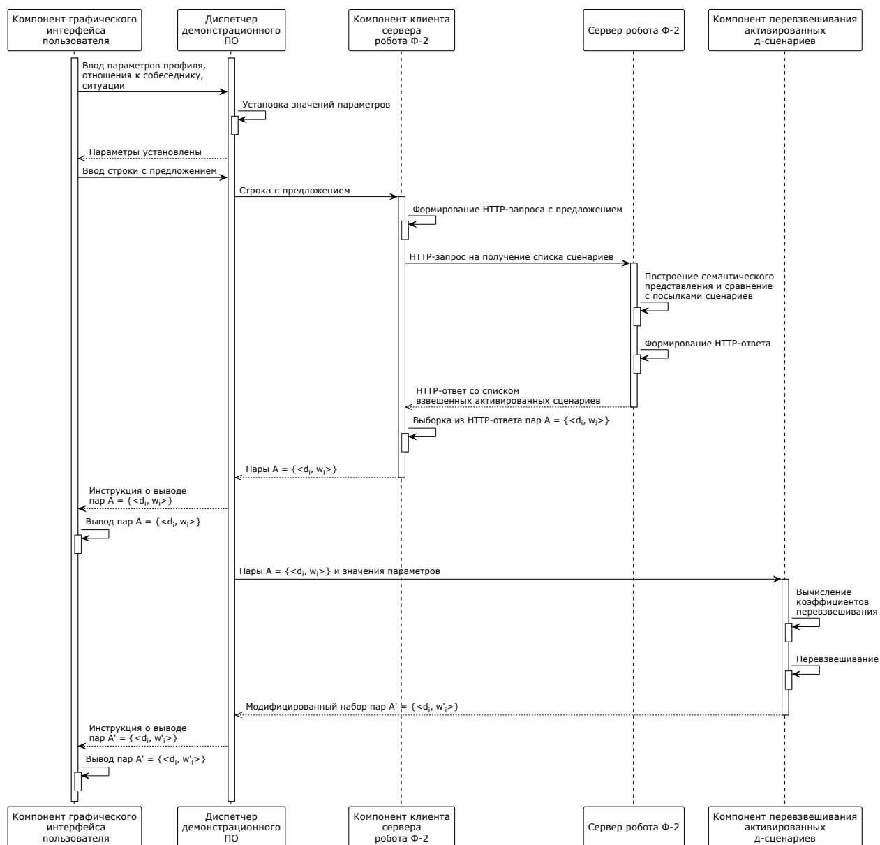
Рисунок 2.6 – Диаграмма последовательностей взаимодействия компонентов блока АЗ с внешними компонентами робота Ф-2
