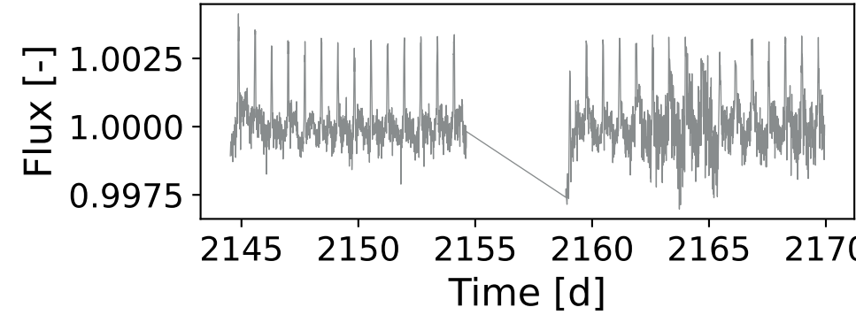
DR3 5168647176826954880 | Sector 31
