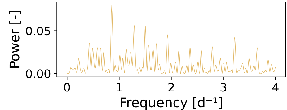
Periodogram < 4 d -1
