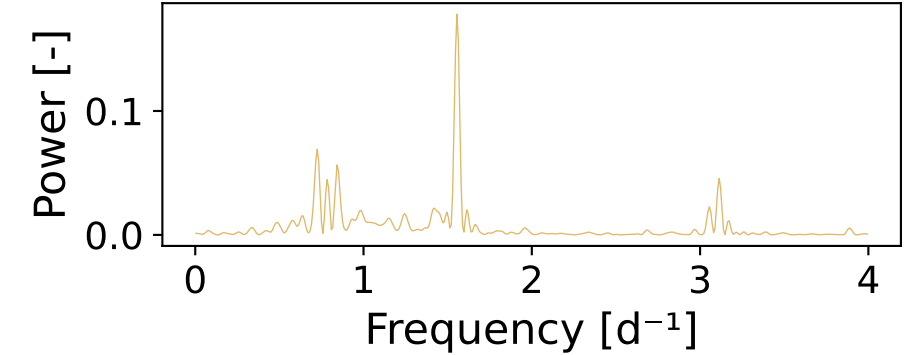
Periodogram < 4 d -1
