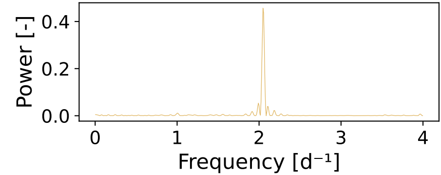
Periodogram < 4 d -1
