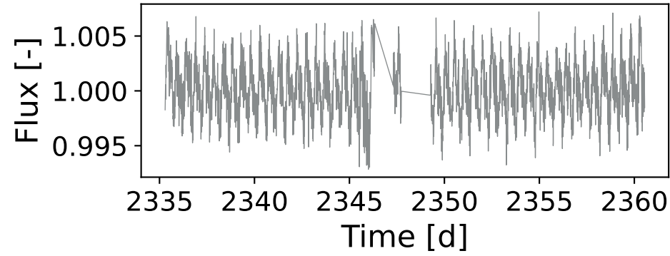
DR3 4657060526856794496 | Sector 38
