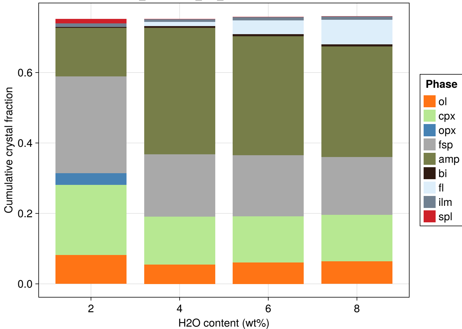
FCX_Cascades_CA_Basalt 4 kbar 1dQFM
