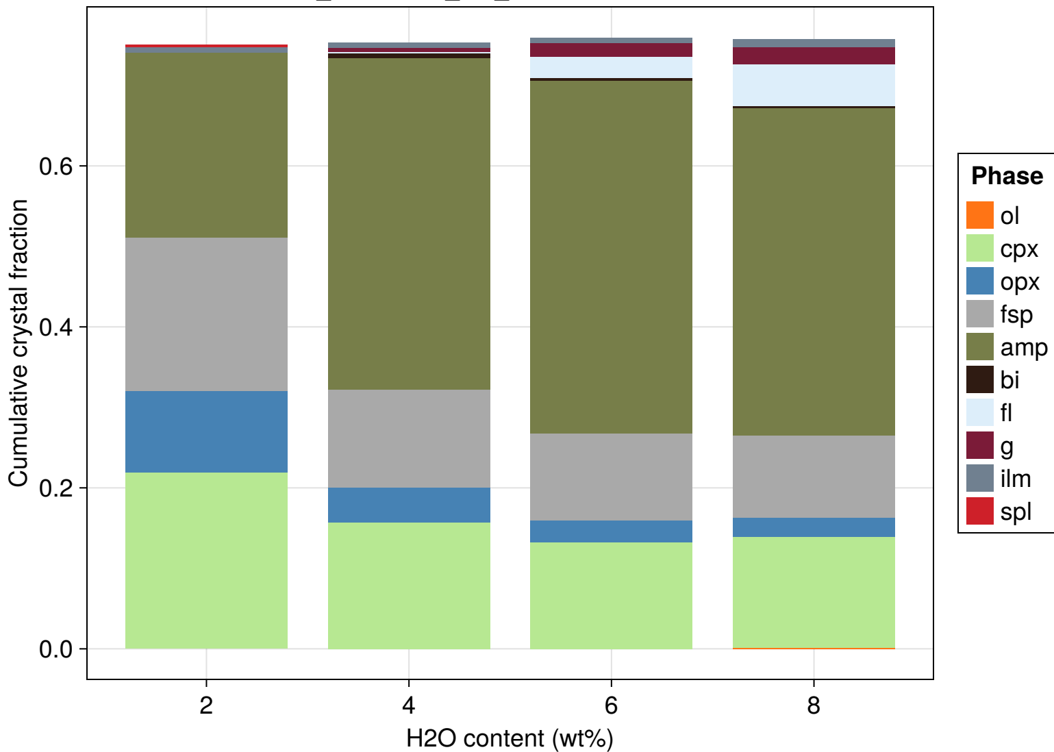
FCX_Cascades_CA_Basalt 7 kbar 1dQFM
