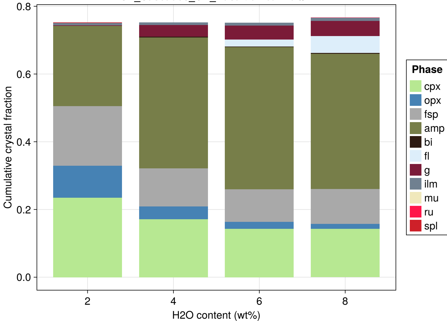
FCX_Cascades_CA_Basalt 9 kbar 1dQFM
