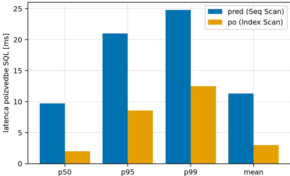
Vpliv sestavljenega indeksa na latenco poizvedbe
