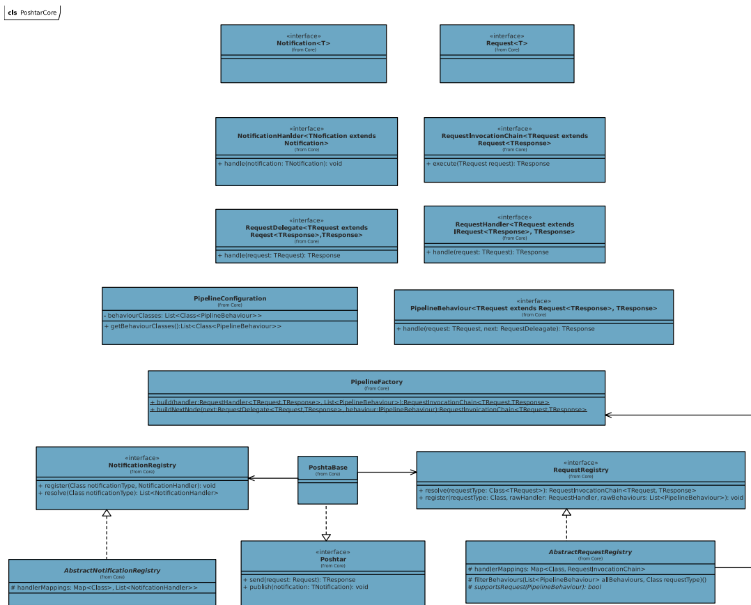
Figure 1: Класни дијаграм језгра библиотеке PoshtaR
