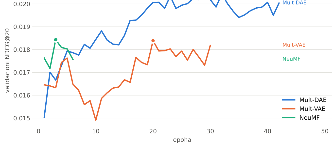
Rano zaustavljanje po validacionom NDCG@20
