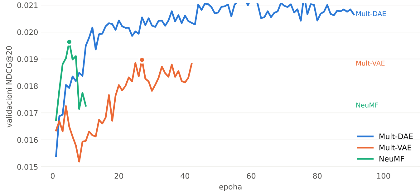
Rano zaustavljanje po validacionom NDCG@20
