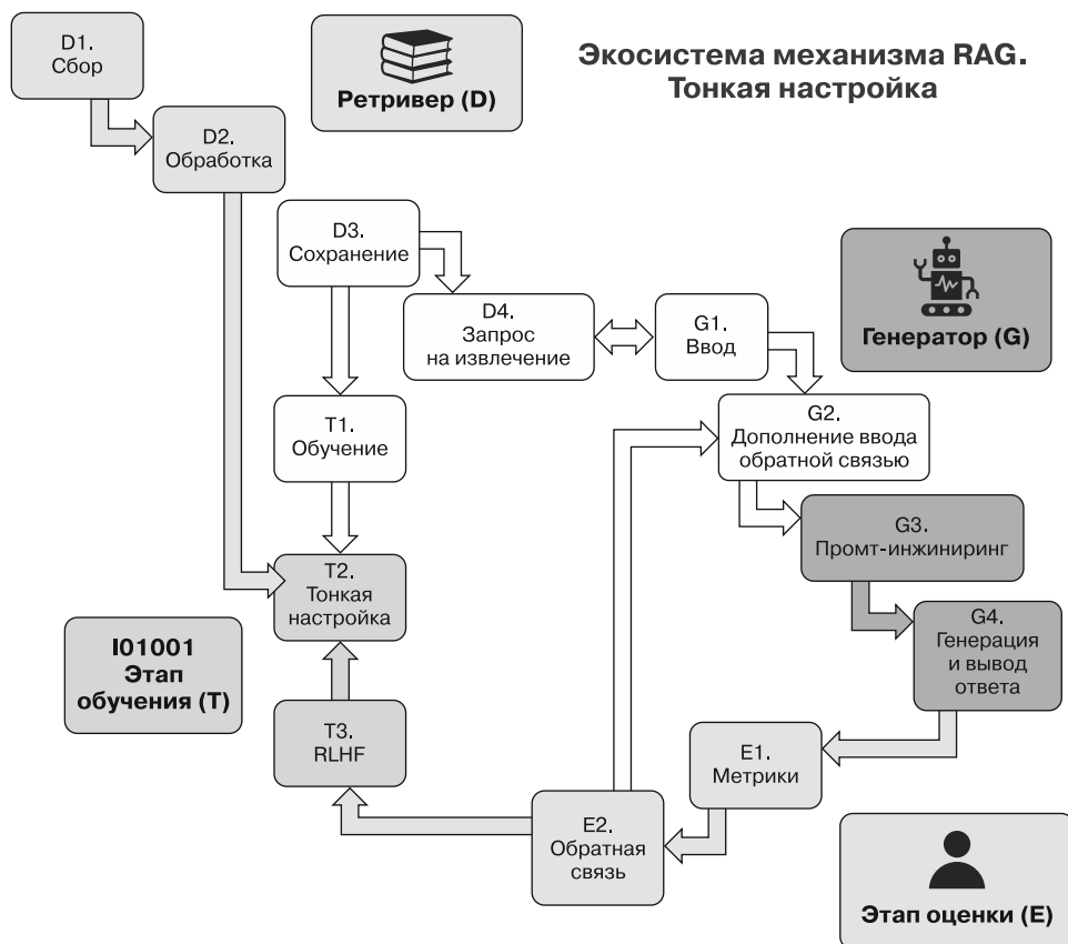
Рис. 9.2. Компоненты тонкой настройки в экосистеме RAG
