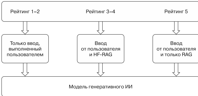
Рис. 5.2. Срабатывание различных вариантов RAG
