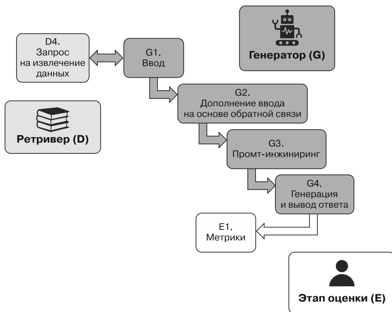
Рис. 4.1. Мультимодальная система RAG
