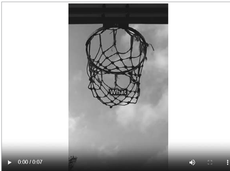
Рис. 10.8. Кадр видео
