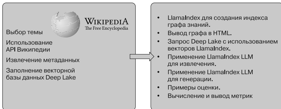
Рис. 7.1. От темы Википедии к взаимодействию с индексом векторной базы данных на основе графа знаний
