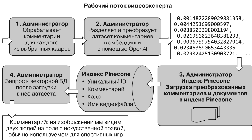
Рис. 10.7. Рабочий поток администратора векторной базы данных от обработки комментариев до их запроса из БД
