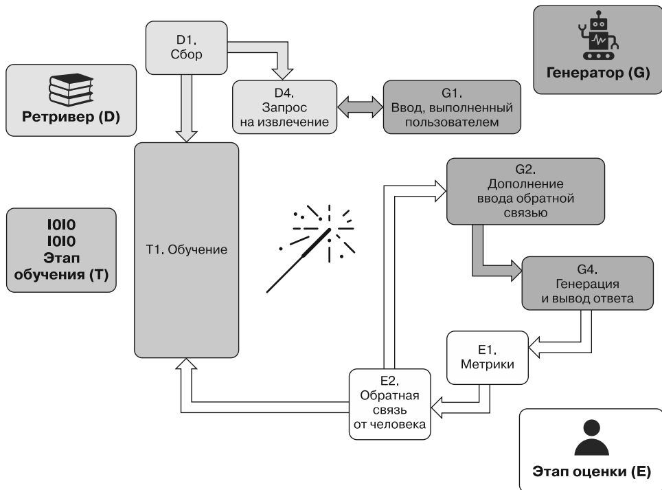
Рис. 5.1. Вариант экосистемы адаптивной RAG
