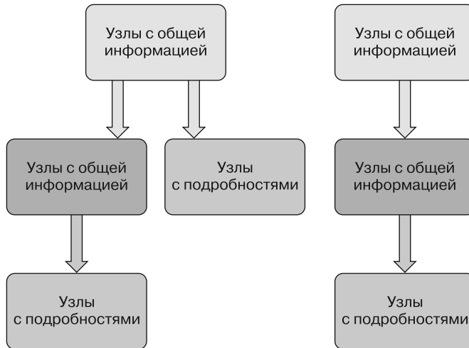
Рис. 3.5. Оптимизированный древовидный индекс
