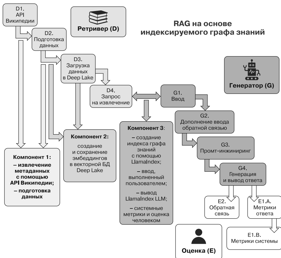
Рис. 7.2. Экосистема графа знаний для RAG
