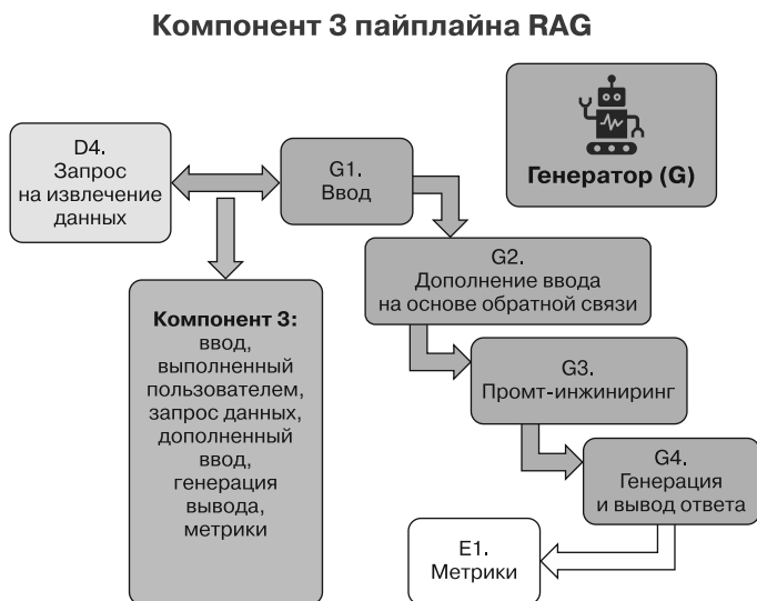
Рис. 2.9. Компонент 3 пайплайна RAG: генерация дополненного ввода
