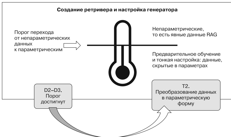
Рис. 9.1. Достижение порога для тонкой настройки данных RAG
