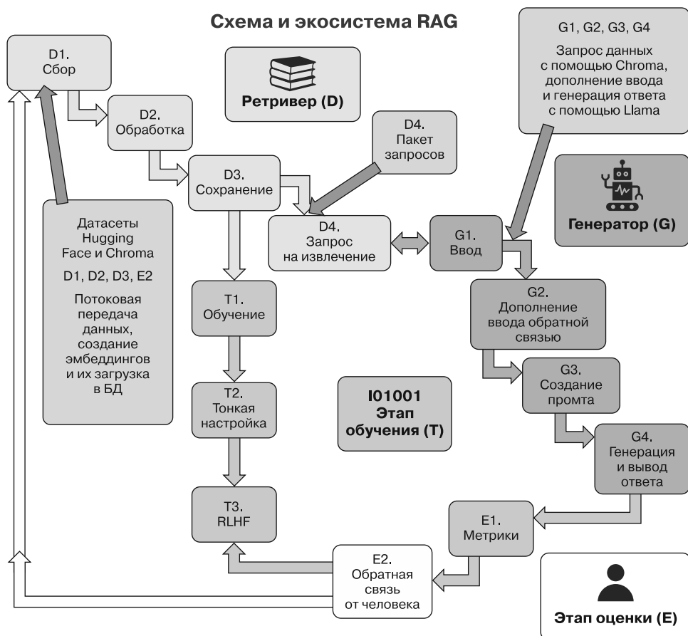
Рис. 8.1. Система динамической RAG
