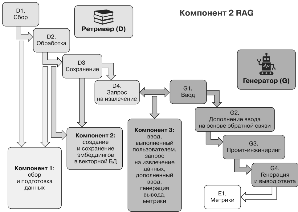
Рис. 2.3. Компоненты пайплайна RAG
