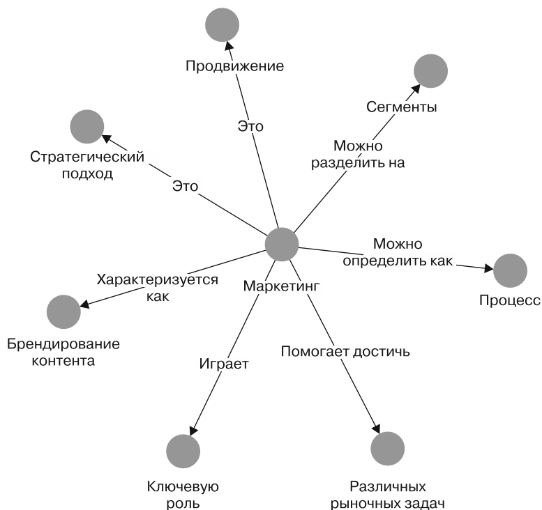
Рис. 7.6. Граф знаний
