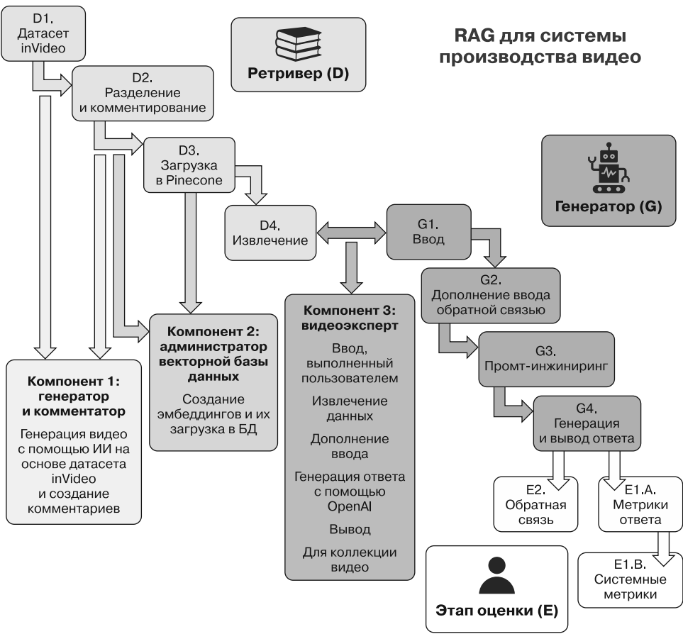
Рис. 10.2. RAG для системы производства видео с использованием агентов генеративного ИИ
