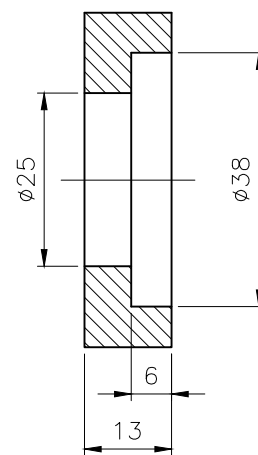
CORTE A-A
