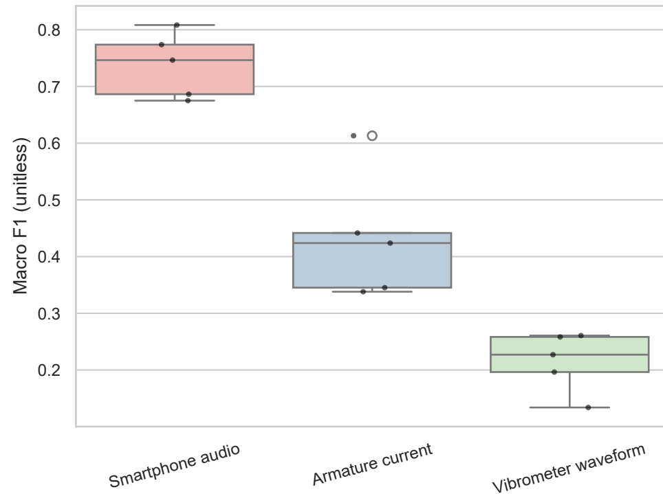
Fold Distribution: Macro F1
