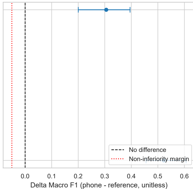
Non-inferiority: Delta Macro F1
