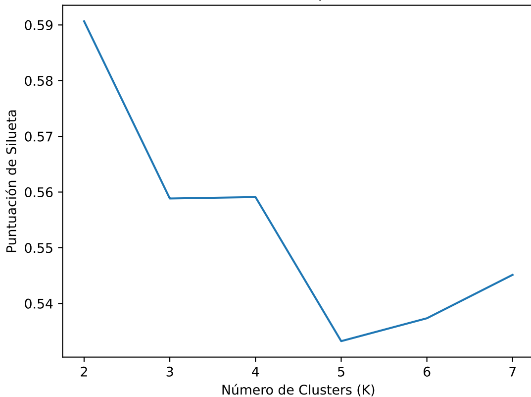
Puntuación de Silueta para Diferentes K
