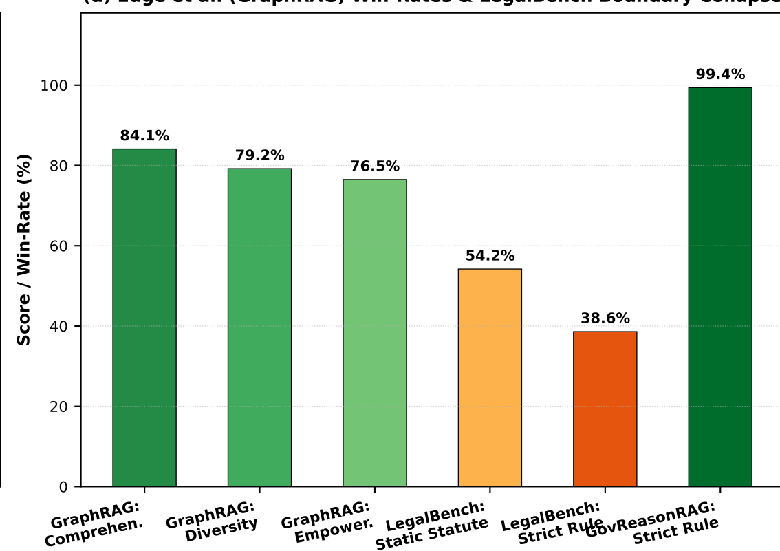
(d) Edge et al. (GraphRAG) Win-Rates & LegalBench Boundary Collapse
